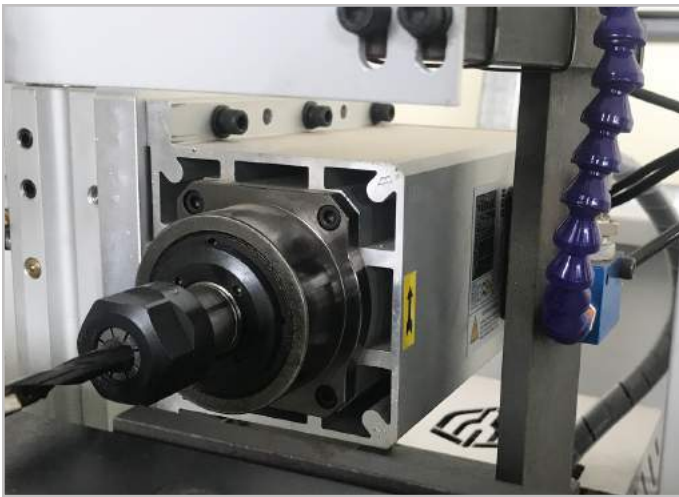
Máy được gia công cao cấp, hệ thống Pad Motor bằng nhôm
