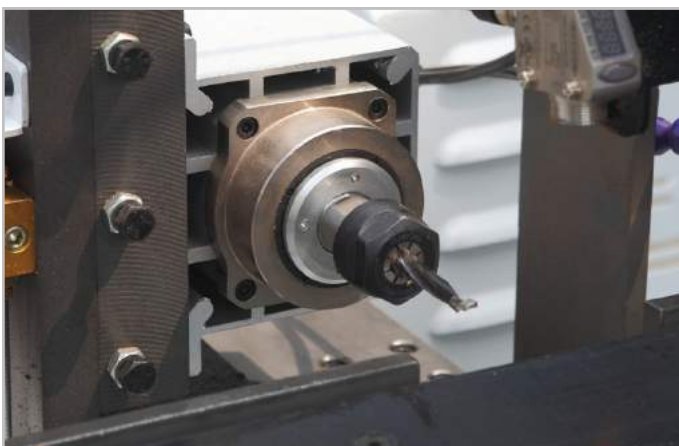
Hai Motor khoan 3,7Kw mạnh mẽ
