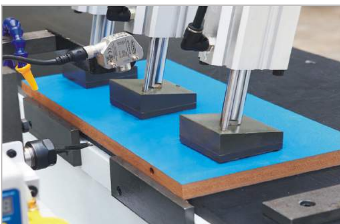
Hệ thống 7 ben kẹp phôi chắc chắn
