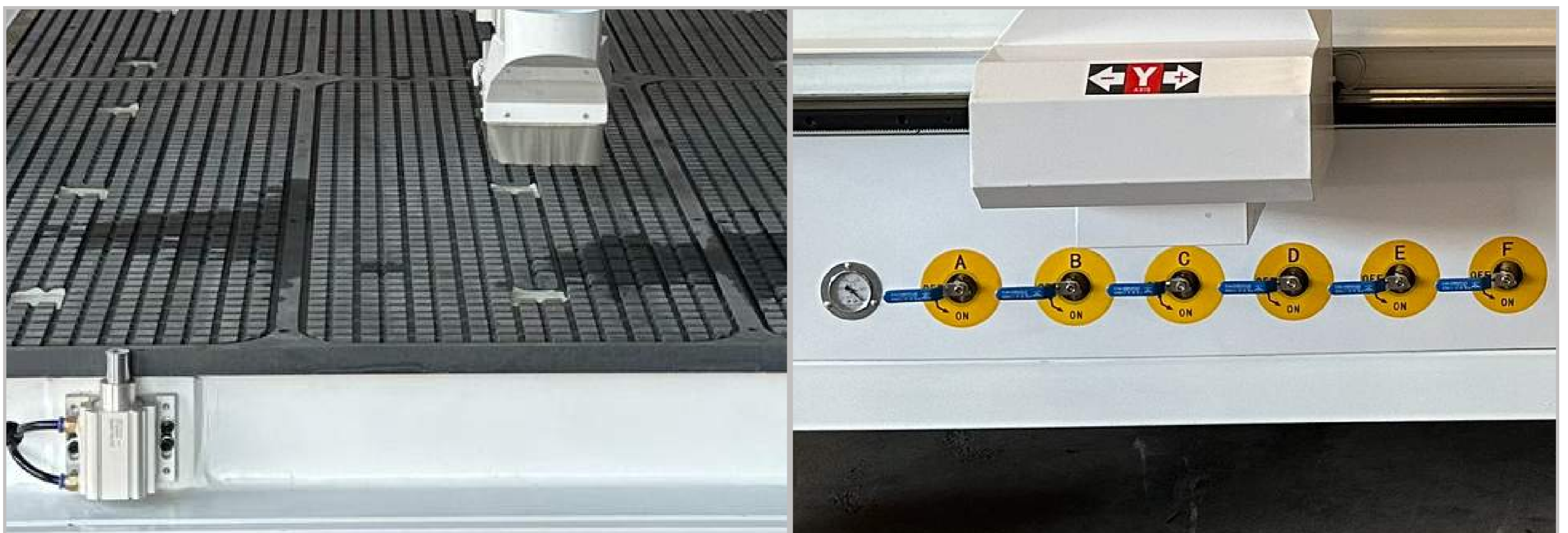
Máy thiết kế tải nặng, bàn hút chân không 6 vùng riêng biệt
