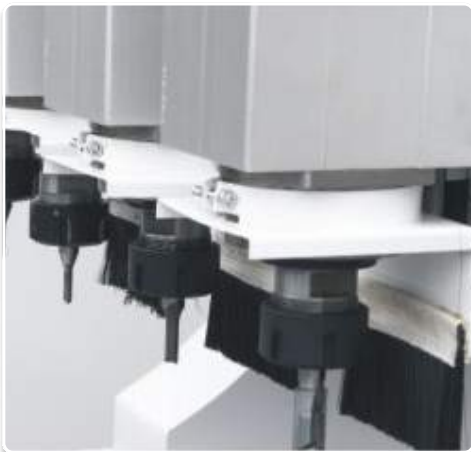
4 đầu Router gia công
