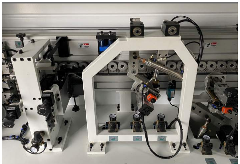
Cạo cạnh 5
