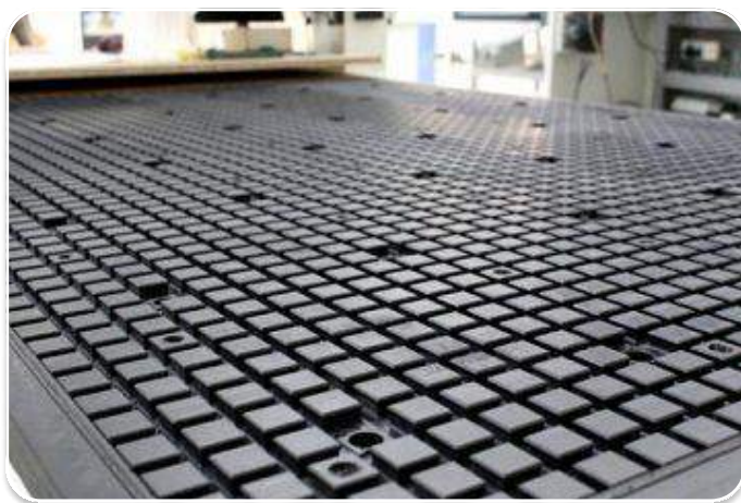
Bàn hút chân không hai lớp lực hút cực mạnh
