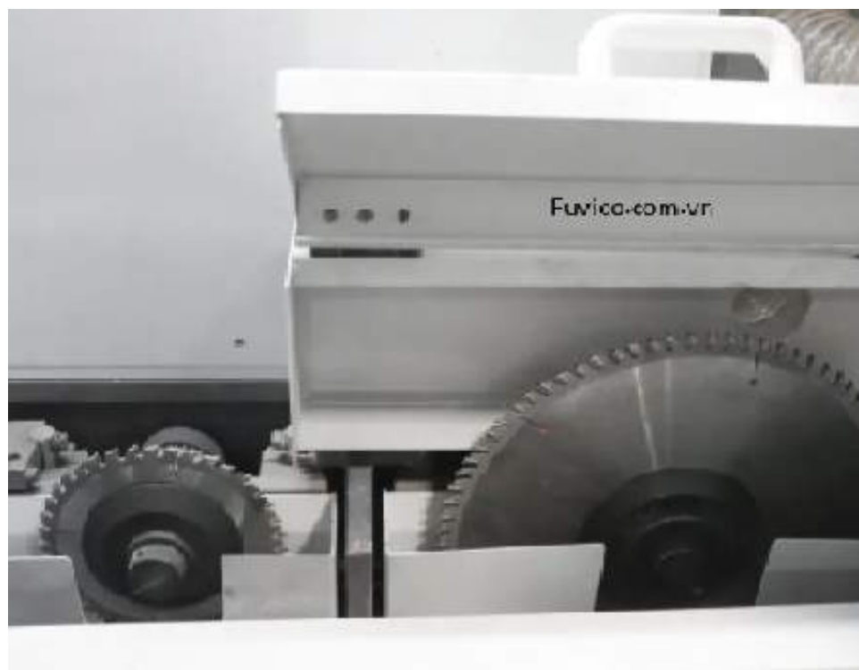
Cụm motor cắt tốc độ cao
