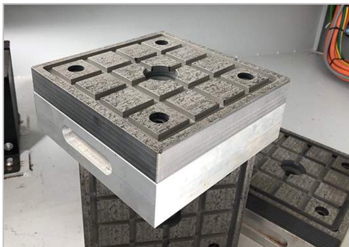
Cục hít ván kê cao đi kèm
