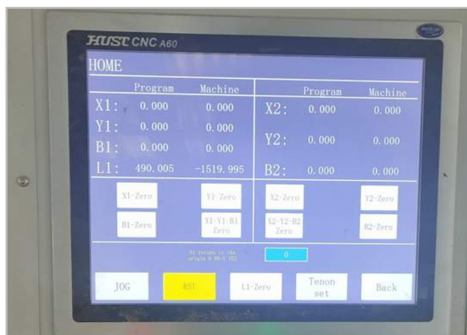
Điều chỉnh thông số mộng cnc trên màn hình
