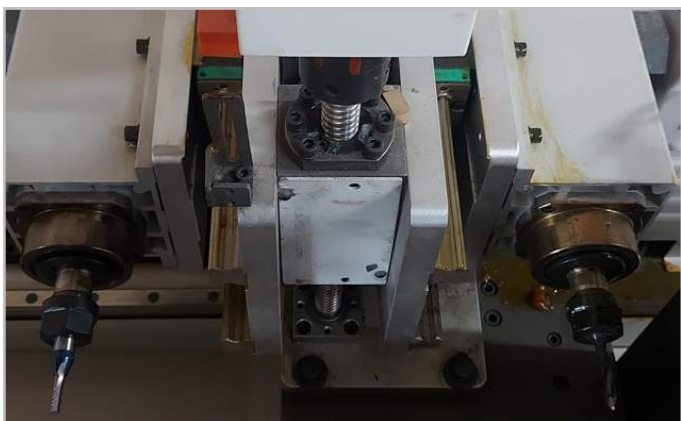
Hai Motor khoan 3,7Kw mạnh mẽ
