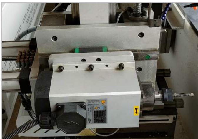
Máy được gia công cao cấp, tải nặng, hệ thống Pad Motor bằng nhôm
