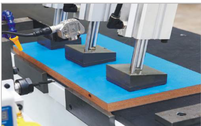
Hệ thống 7 ben kẹp phôi chắc chắn
